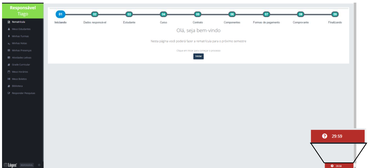
Figura 1: Página Inicial
