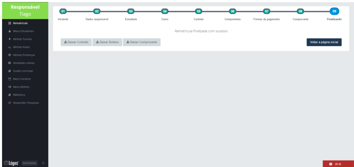
Figura 10: Reimprimindo
